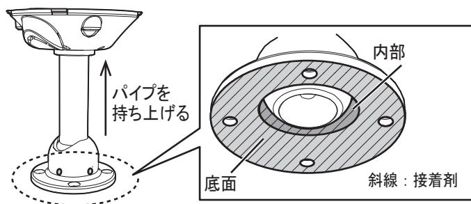
直型アンテナベースの土台
